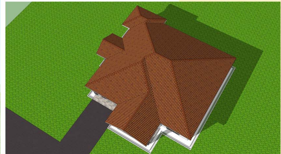
DESIGN D129 Banglo Setingkat 5 bilik/3 bilik air 2370kaki persegi
